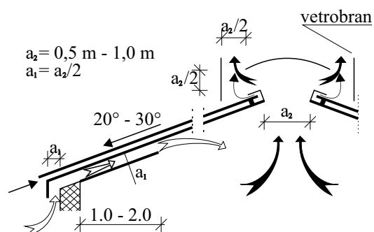
Slika 12. Detalj proračuna kanala i lanterne
