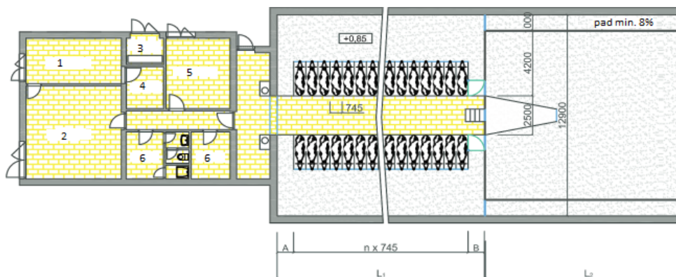
Slika 16. Paralelno izmuzište
